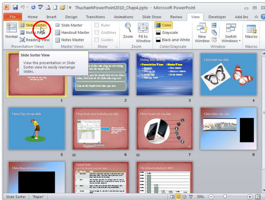
Hình 304. Slide Sorter
